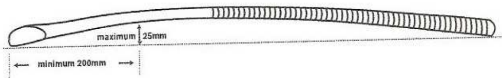
Figura 6: Dispositivo para medir el arco o inclinación del palo
